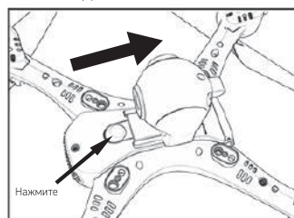
ДЕМОНТАЖ КАМЕРЫ
